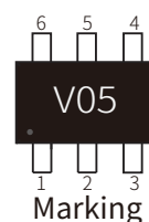
SOT-23-6L
